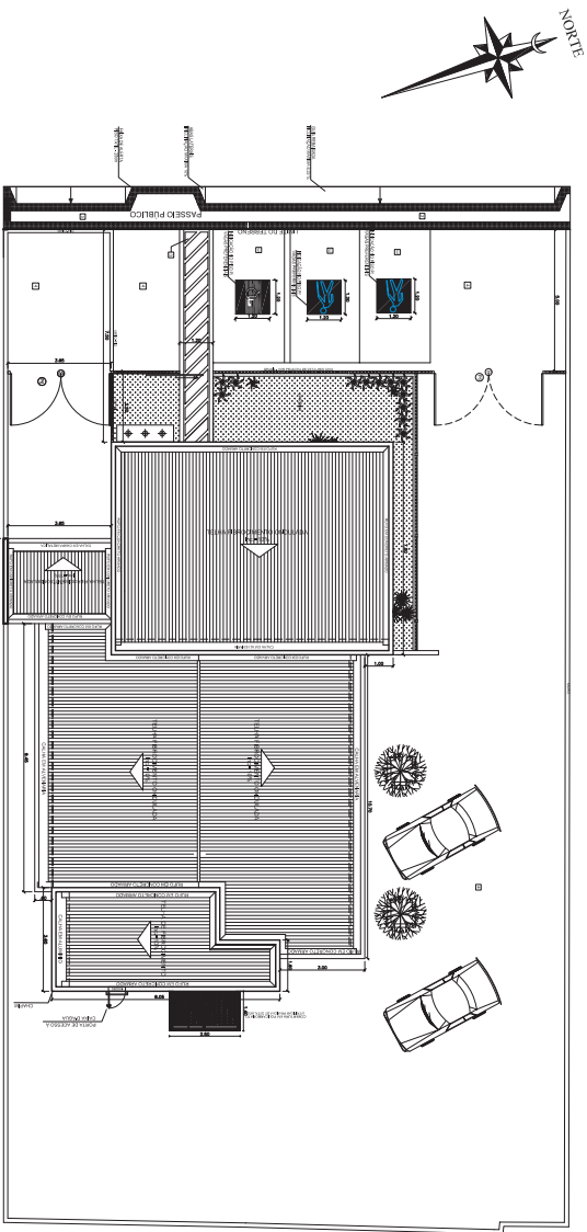
PLANTA DE COBERTURA E ACESSIBILIDADE ESCALA 1/100
