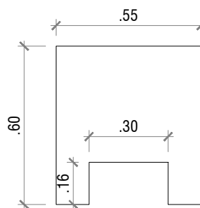
VISTA LATERAL ESCALA 1/20
