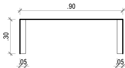
VISTA SUPERIOR ESCALA 1/20
