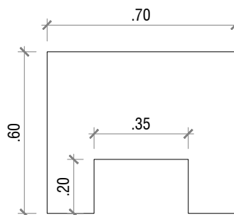
VISTA LATERAL ESCALA 1/20
